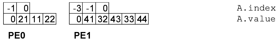
図 11: DIA 形式のデータ構造 (マルチプロセス環境)
